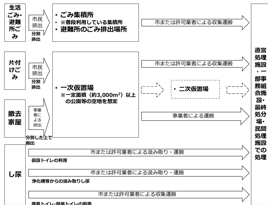
災害時に発生する廃棄物の処理の流れ（案）
