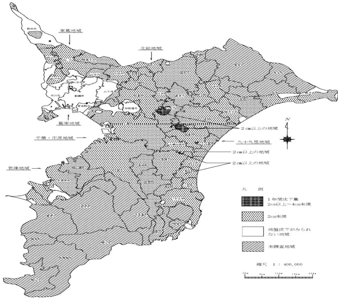
図6-2 千葉県水準基標変動図(1年間変動図) (平成21年1月～平成22年1月)
