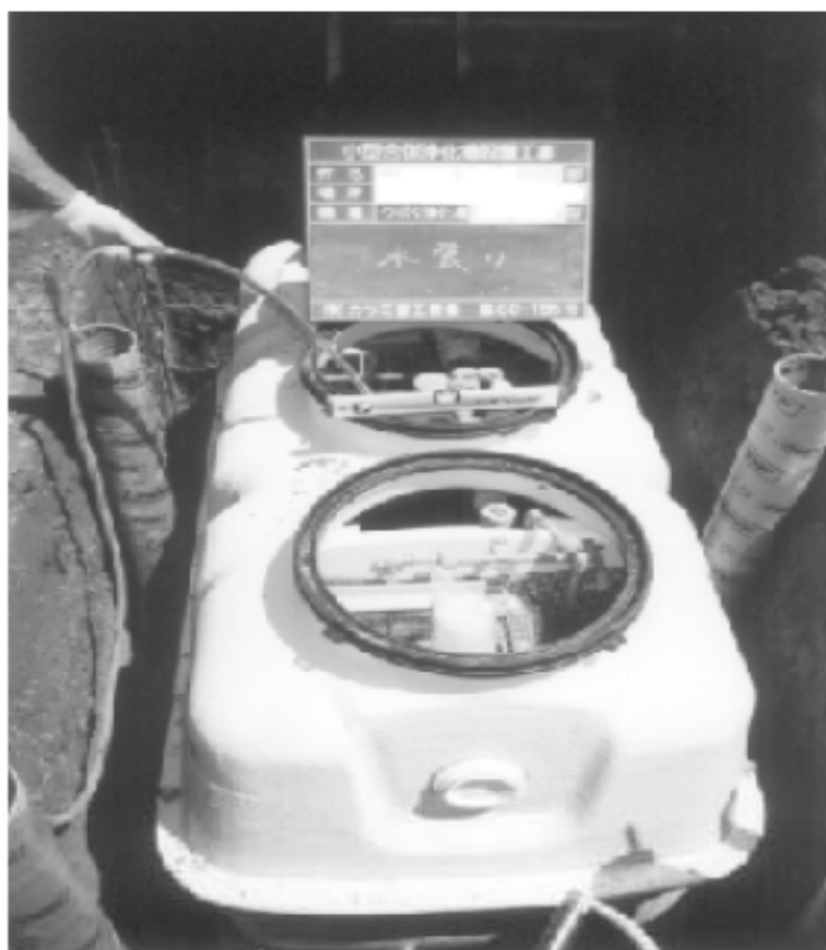
家庭用小型合併処理浄化槽
