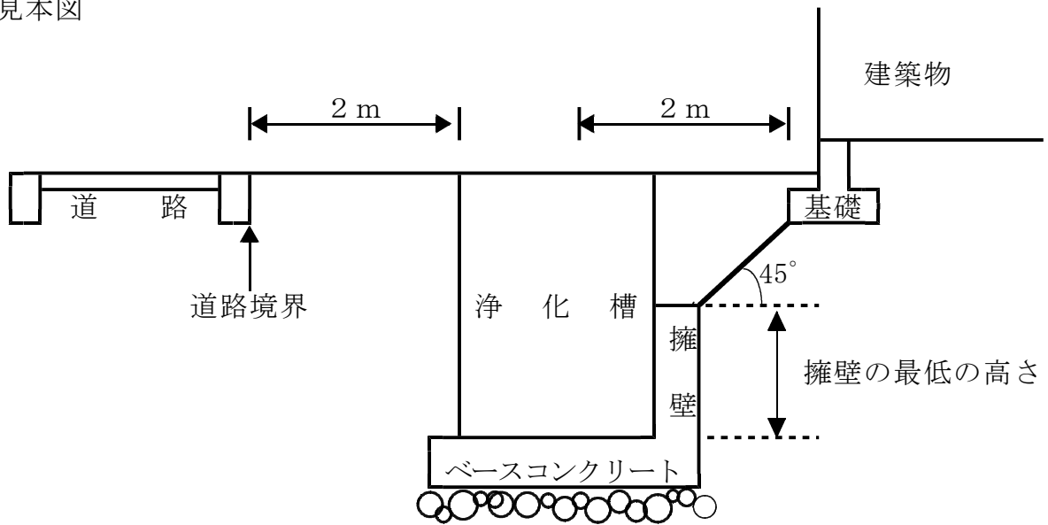
擁壁見本図
