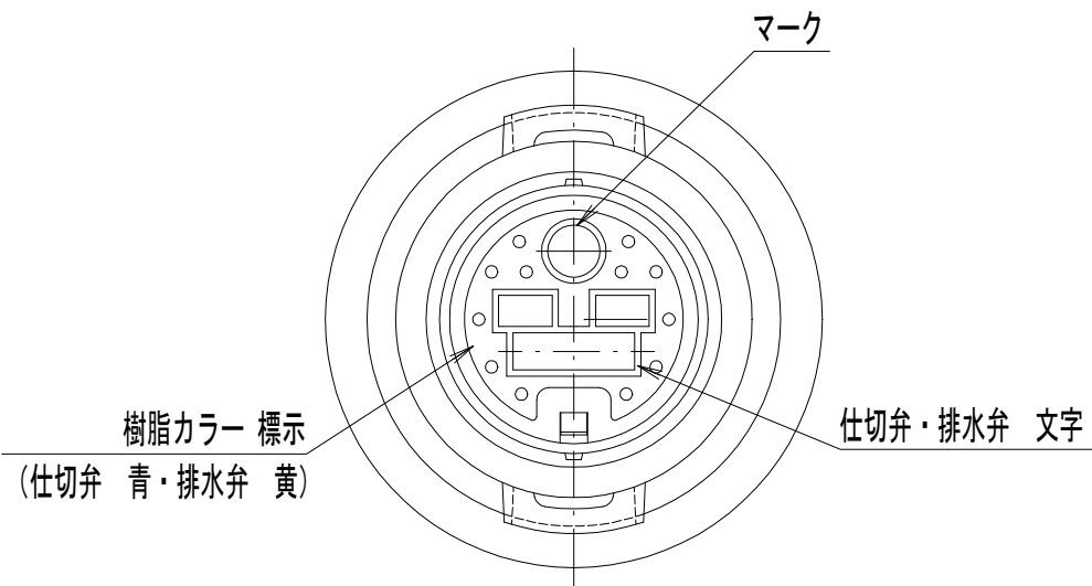
平面図
