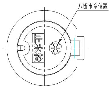
蓋，ホルダー平面図
